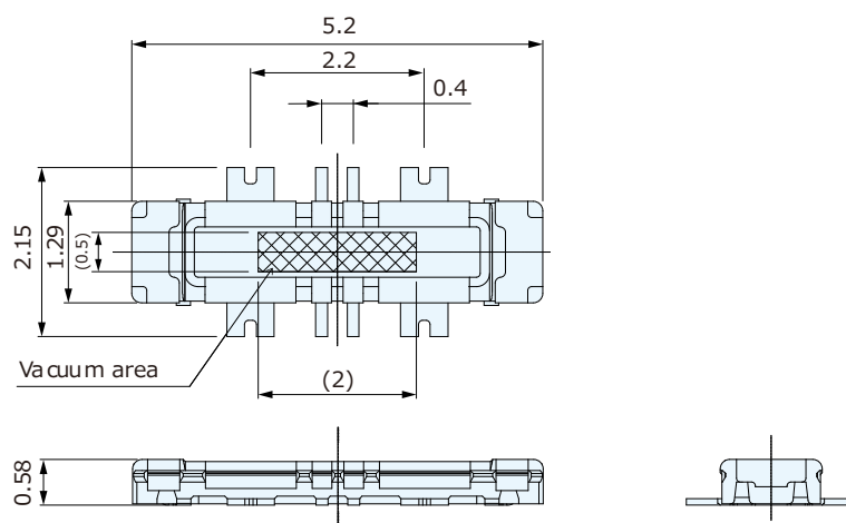
プラグ : CPBE208-0101F
