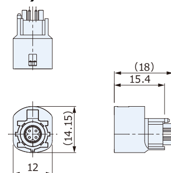
プラグ(バーチカルタイプ) : CSC5004-6C□□F
