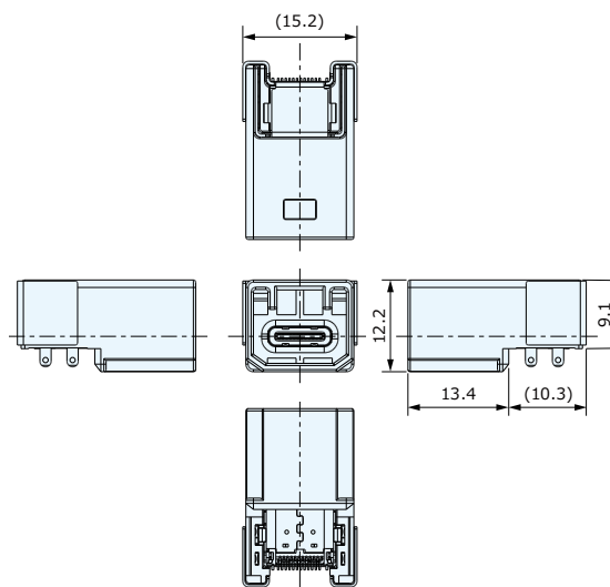
Cable Plug : CSC1024-4J□□F
