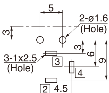
取付基板参考図(パターン側)・適合プラグ
