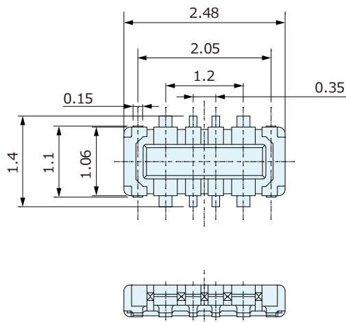
プラグ : CPBD408-0101F
