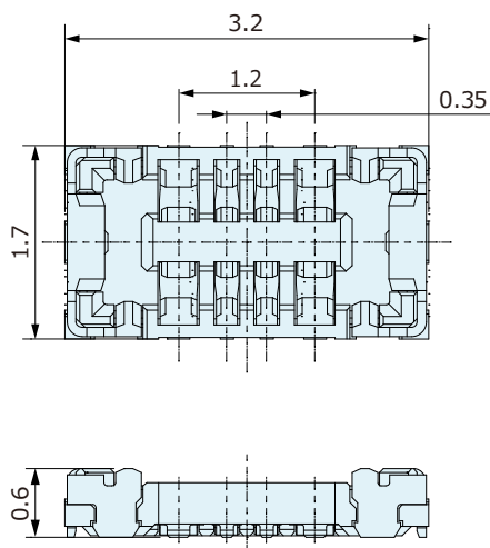
プラグ : CPBD408-0101F
