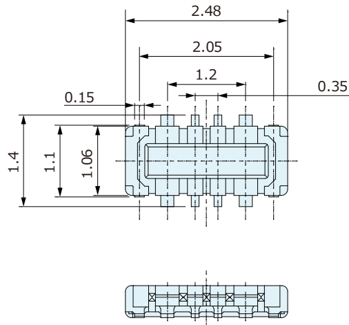
プラグ : CPBD408-0101F
