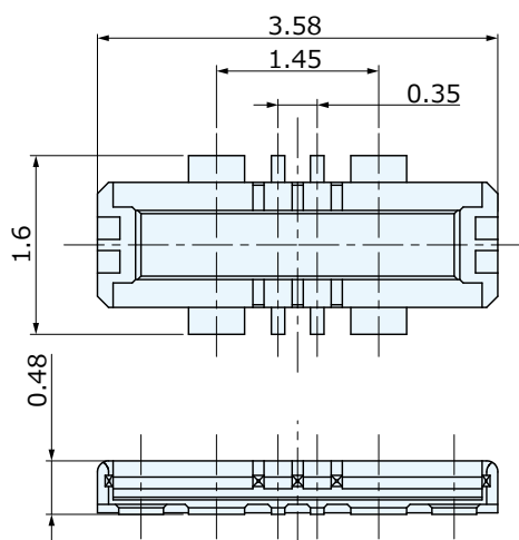
Plug : CPBF408-0101F
