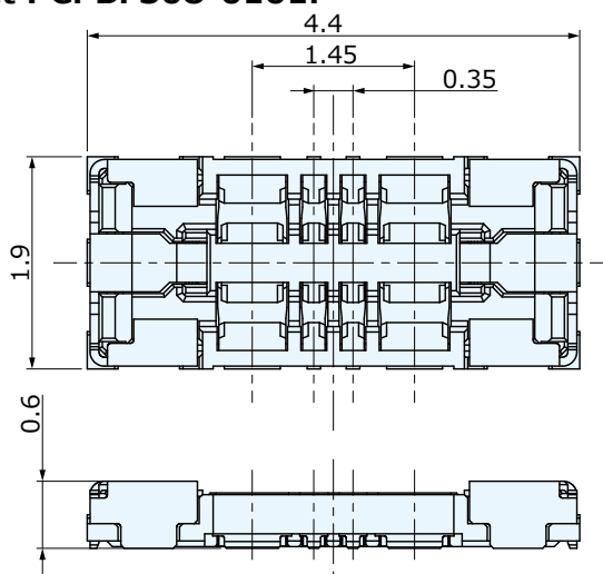
Socket : CPBF308-0101F
