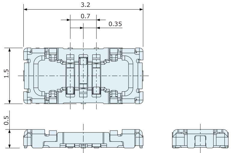
プラグ : CPBE405-0101F
