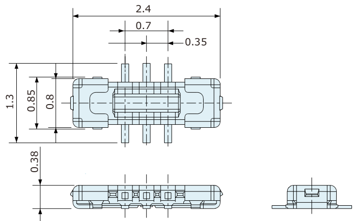
プラグ : CPBE405-0101F
