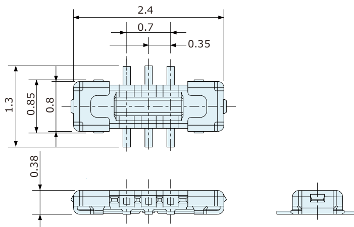
プラグ : CPBE405-0101F
