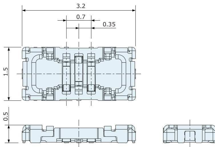
プラグ : CPBE405-0101F
