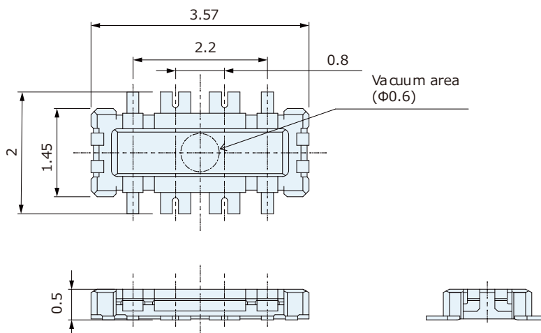
プラグ : CPBA306-0101F
