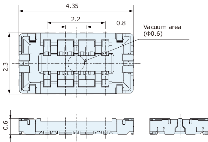
プラグ : CPBA306-0101F
