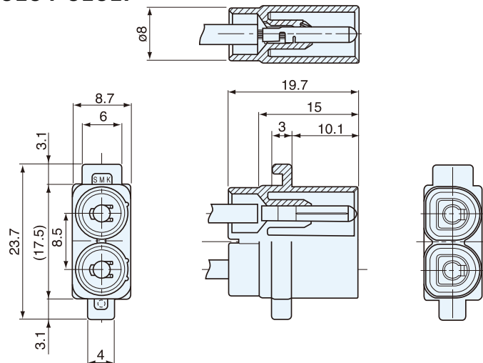
プラグ : CCT0104-0101F
