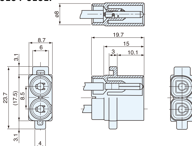
プラグ : CCT0104-0101F
