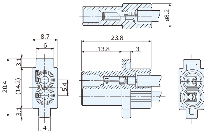
ソケット : CCL0505-0120F
