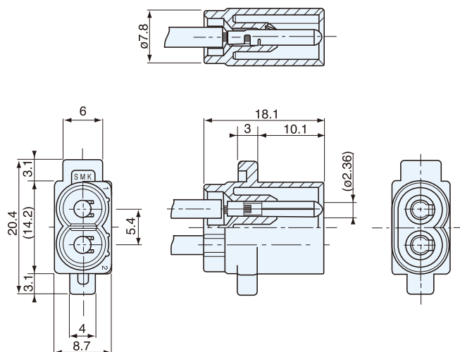
プラグ : CCL0105-0100F
