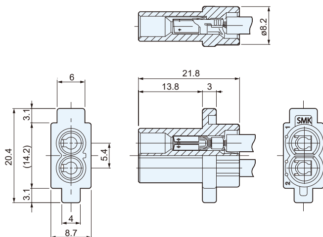
ソケット : CCL0505-0100F
