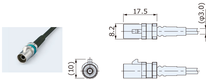
电缆插头(防水) CRC1001-57□□F
