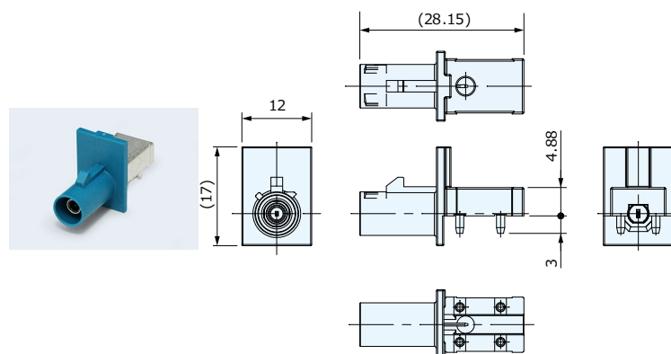
基板用Plug (破板型・防水) CRC5001-74□□F
