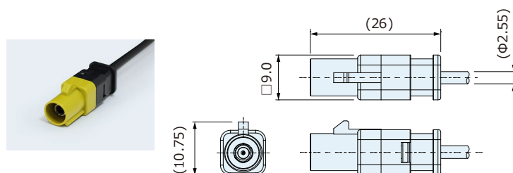
电缆插头(旋转) CRC1001-56□□F
