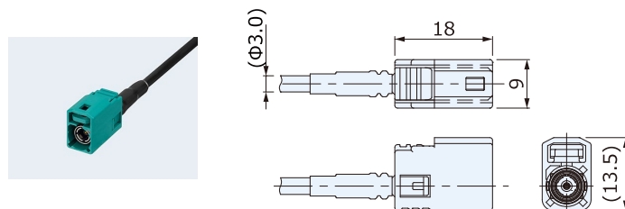
电缆插孔(防水) CRS9001-45□□F
