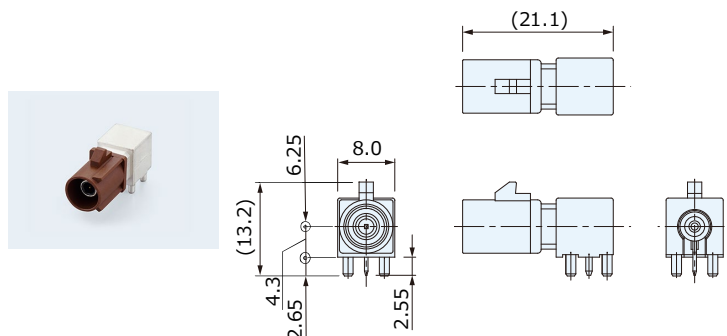
基板用Plug CRC5001-70□□F
