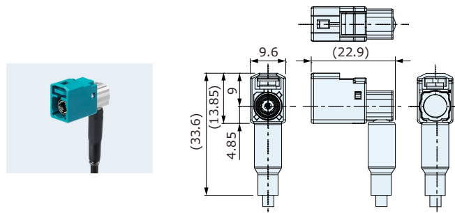
电缆插孔(防水) CRS9001-46□□F
