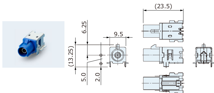
基板用Plug CRC5001-58□□F
