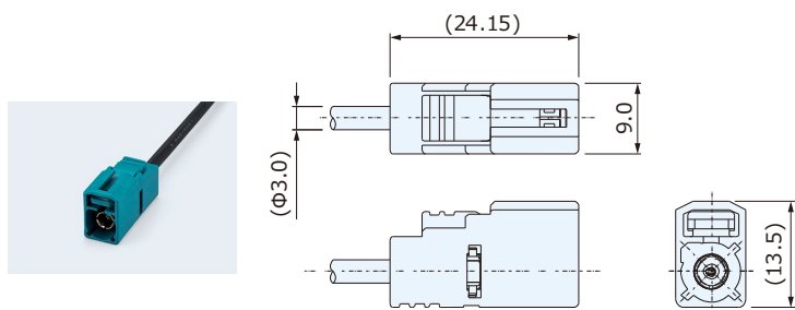
电缆插孔 CRS9001-23□□F
