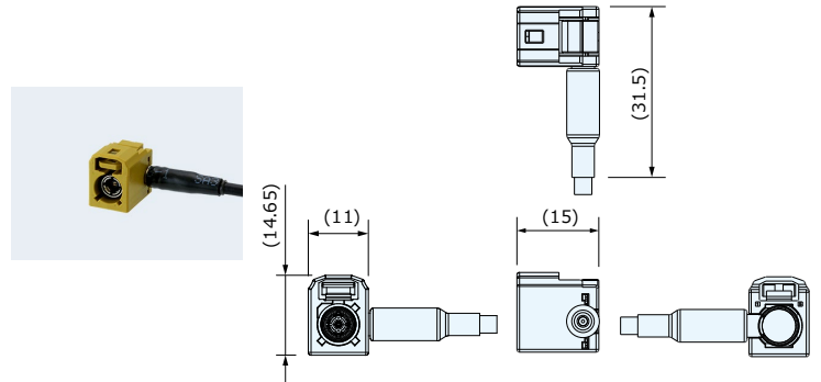
电缆插孔（低背・防水） CZF2100-03□□F
