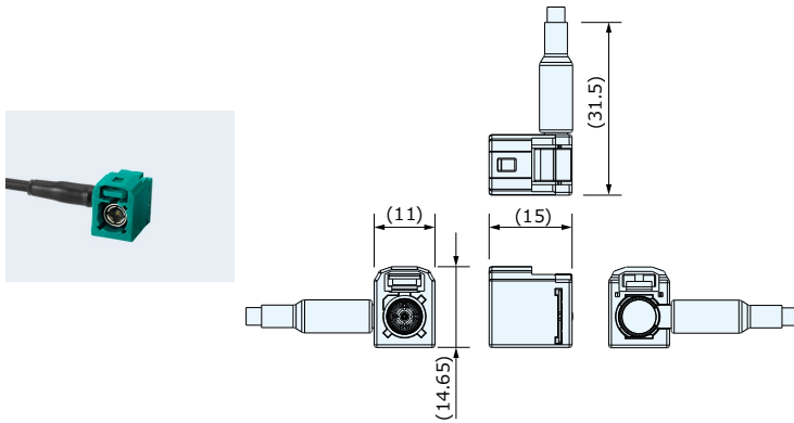
电缆插孔（低背・防水） CZF2100-02□□F
