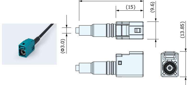
电缆插孔(防水・旋转) CRS9001-38□□F
