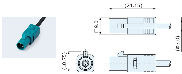
电缆插头 CRC1001-52□□F
