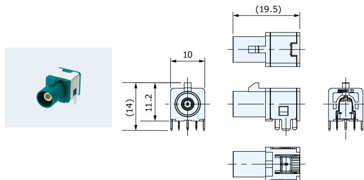
基板用Plug CRC5001-90□□F
