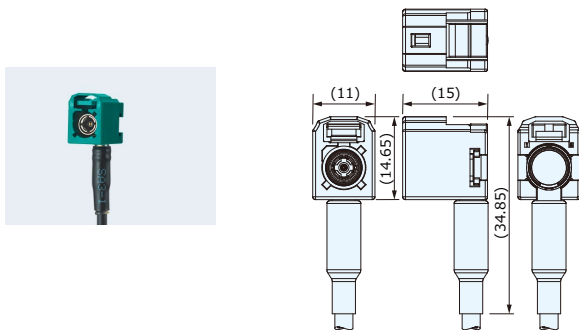
电缆插孔（低背・防水） CZF2100-13□□F
